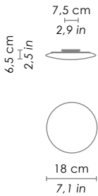
Versione da incasso con alimentatore in remoto version with recessed remote power adaptor.
