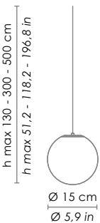
Elemento componibile - gruppo luce modular element - lamp component kit
