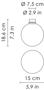
Versione con alimentatore nella base version with power adaptor in the base
